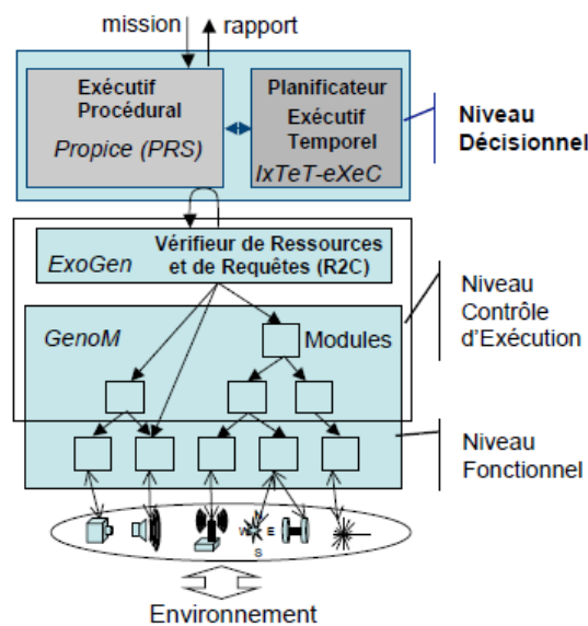
Figure 10 L'architecture LAAS (tiré de [Ingrand, 05])
